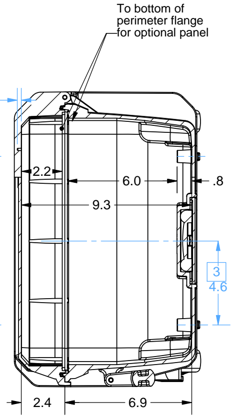
SECTION A-A
