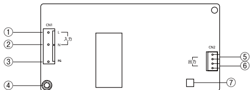
ZWS5部品面
