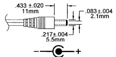
Dim.: mm
