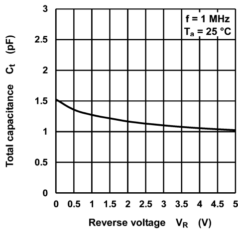
Fig. 8.4 C_t - V_R
