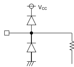
Pin 12 (IS-)
