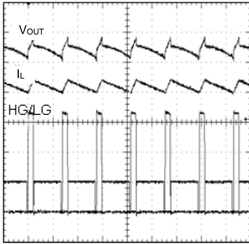
Figure 26. SLLM Mode ( I_{O}=1A )
