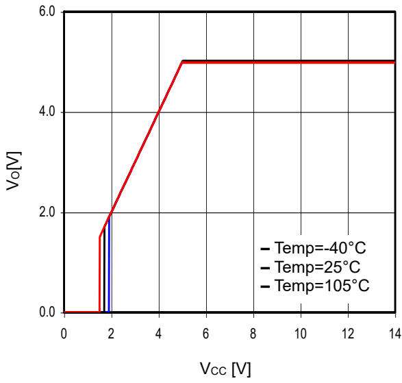
Fig. 27 V_{cc}-V_o ( I_o=0\text{mA} )
