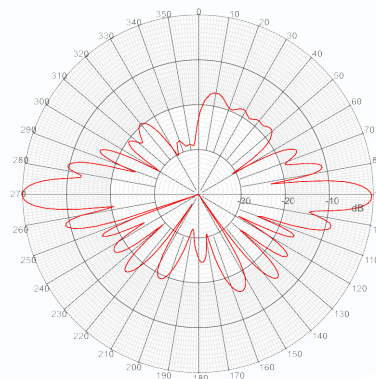
E-plane 3.55 GHz
