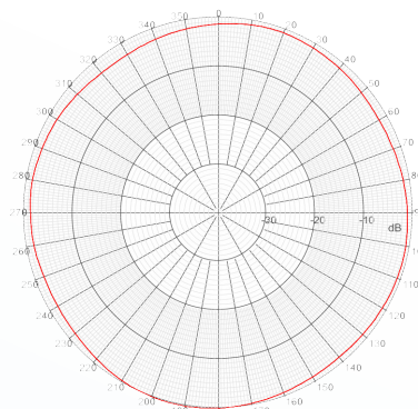
H-plane 3.55 GHz
