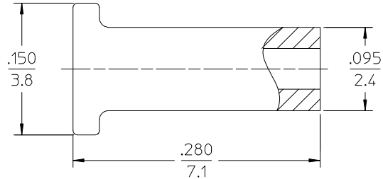
DUST CAP
