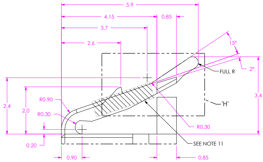
DETAIL 'G' SCALE 12:1
