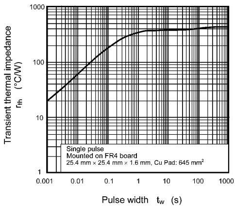
Fig. 7.11 r_{th} - t_w
