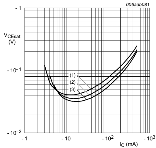
I_C/I_B = 50 (1) T_{amb} = 100^\circ C (2) T_{amb} = 25^\circ C (3) T_{amb} = -40^\circ C
