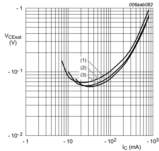
I_C/I_B = 100 (1) T_{amb} = 100^\circ C (2) T_{amb} = 25^\circ C (3) T_{amb} = -40^\circ C
