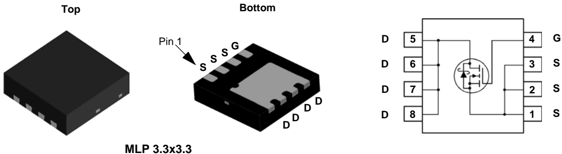
MLP 3.3x3.3
